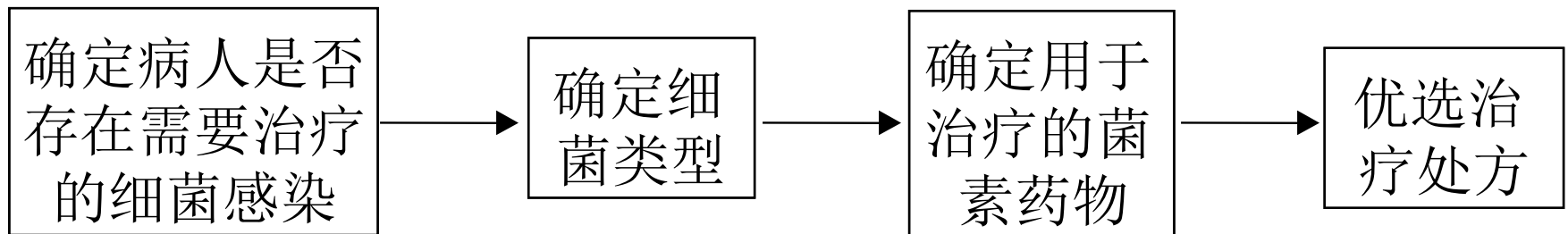
MYCIN系统的咨询过程
