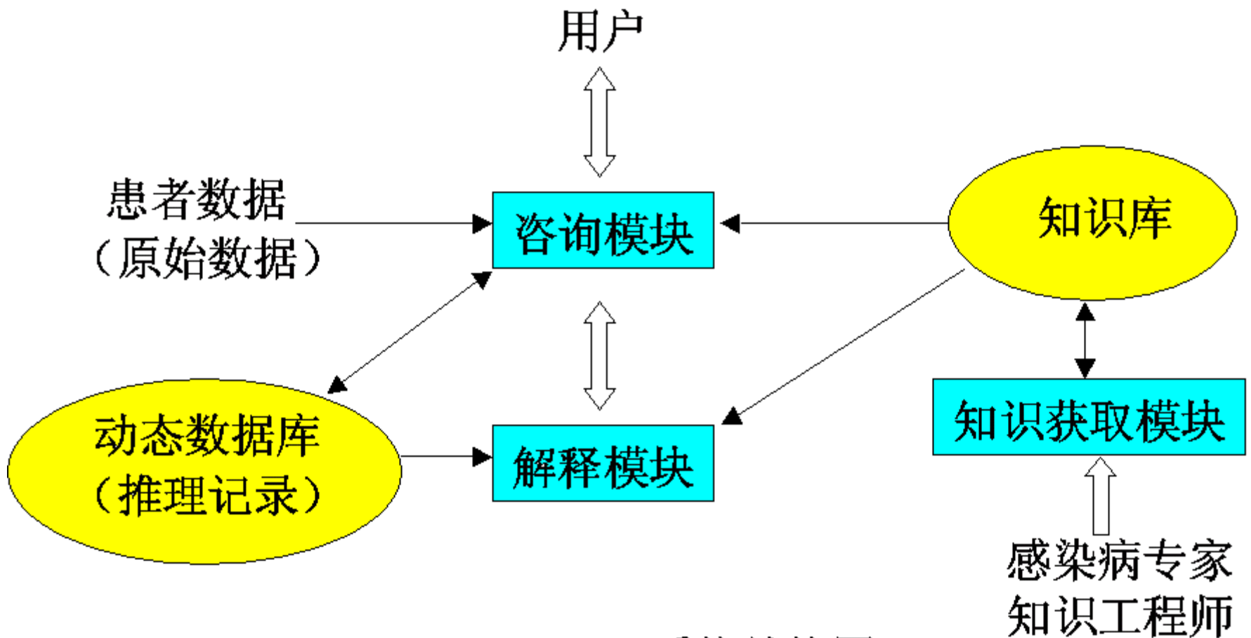
MYCIN系统结构图
